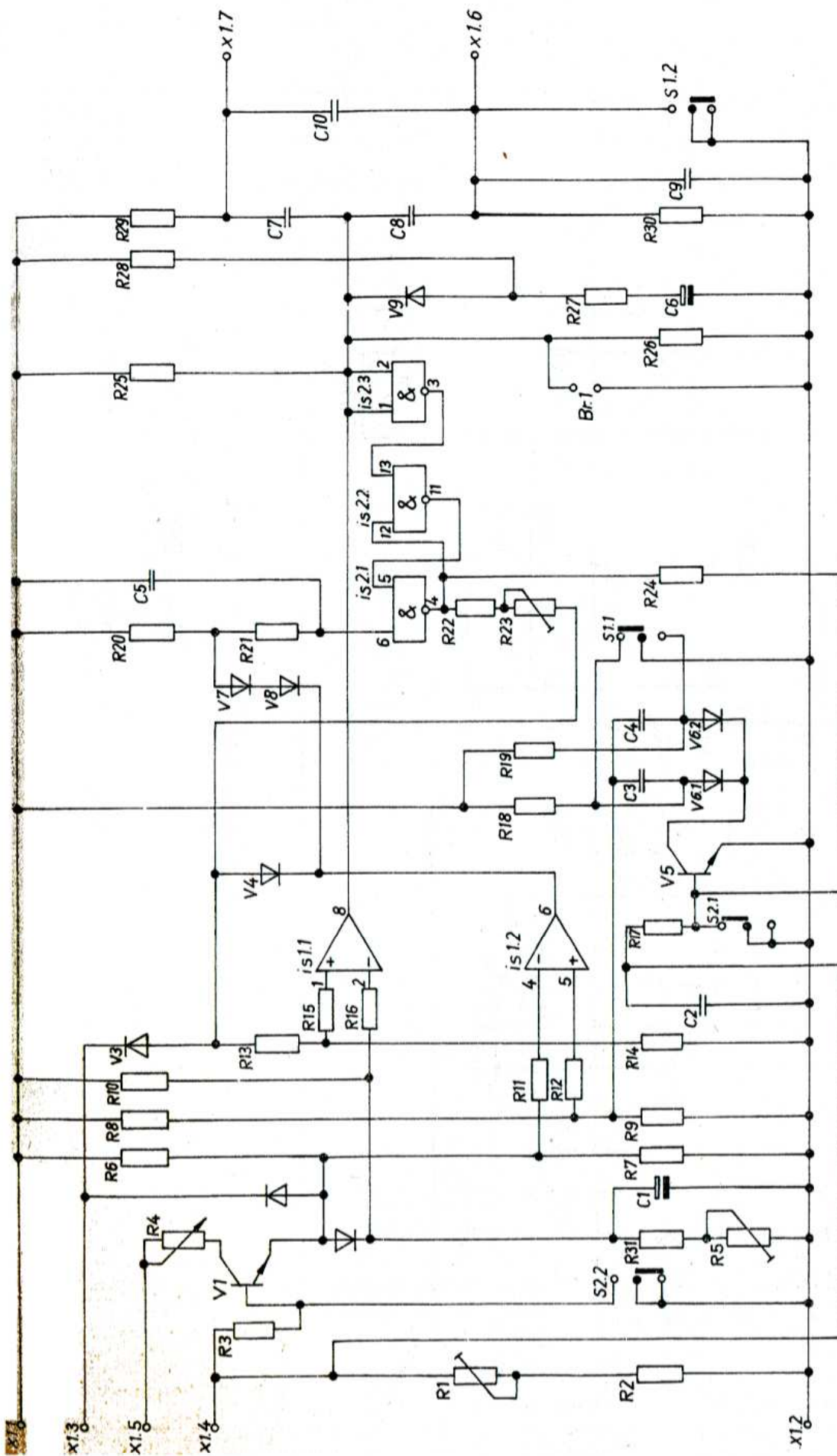
Stromlaufplan (Nadelpositionierung) Wiring diagram (needle positioning) Schéma des connexions (positionnement de l'aiguille) Overzicht van het stroomverloop (naaldstandzoeker) План прохождения тока (механизм позиционирования иглы) Plán rozvádění proudu (polohování jehly) Huzalozási vázlat (tűpozicionálás)
