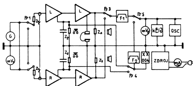
Obr. 3. Zapojení pracoviště pro měření zesilovače
